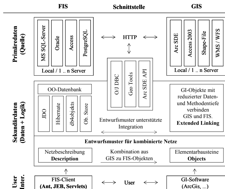
Abbildung 1: Systementwurf der Agricultural-GIS-Sphere
