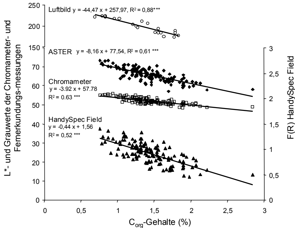
Abbildung 1: Abhängigkeit der optischen Parameter (L*-Werte aus Chromameter-Messungen, Grauwerte aus Luftbild- und aus ASTER-Daten, f(R) nach Kubelka-Munk aus HandySpec Field-Messungen) von den C_{\text{org}} -Gehalten auf dem Testfeld Demmin
